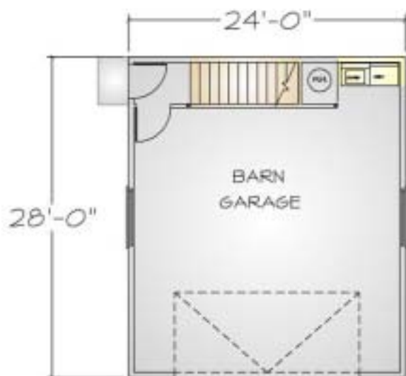
1 階床プラン
